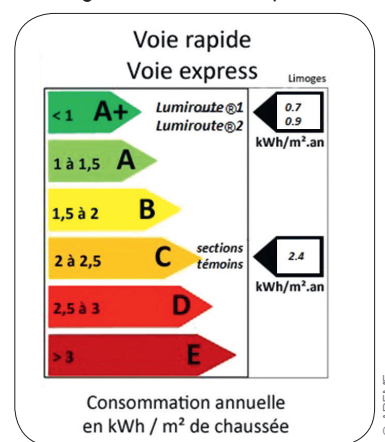
-Figure 6- Étiquette énergie des 4 sections expérimentées.
